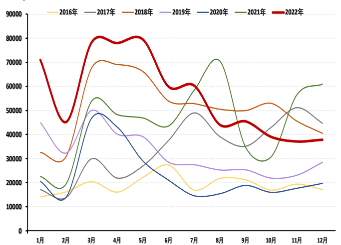
硅铁出口量
