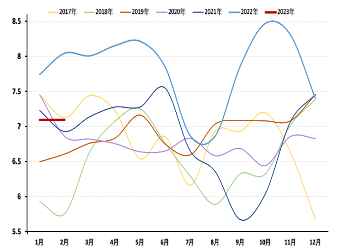
金属镁产量
