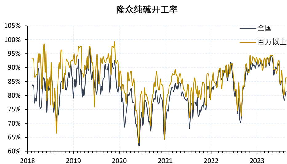
Figure 4 隆众开工率（%）
