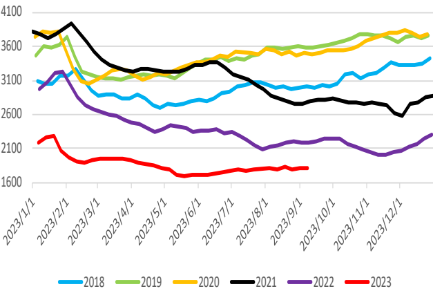
焦煤总库存
